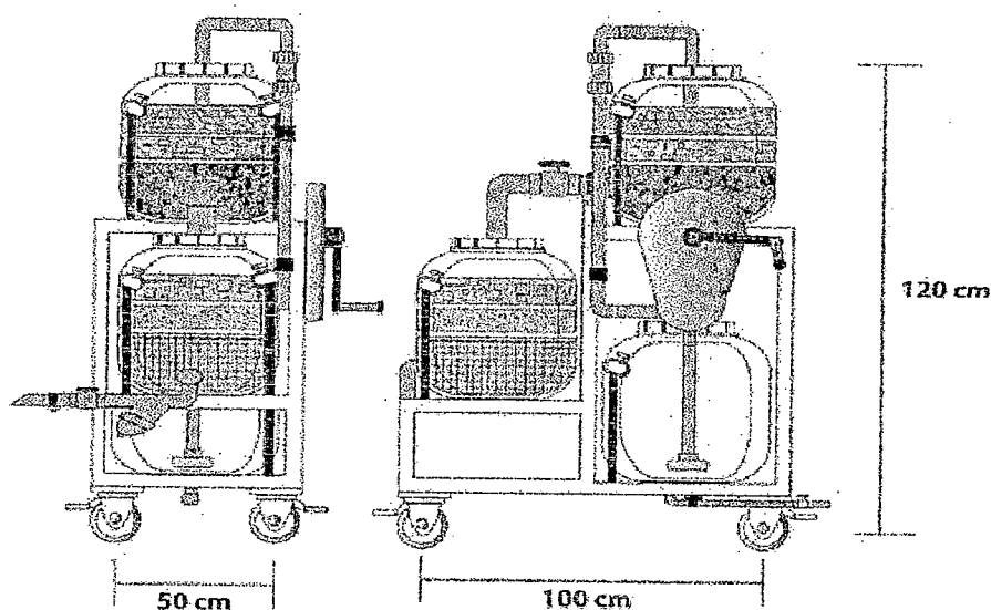
ภาพที่ 1 แบบร่างอุปกรณ์บำบัดน้ำเสียจากกระบวนการย้อมผ้าในชุมชน
